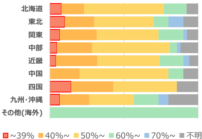
ケージ内の湿度 夏季平均
